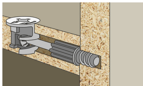
Скрытый крепеж Эксцентрик
