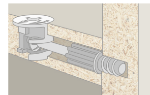
Скрытый крепёж Эксцентрик
