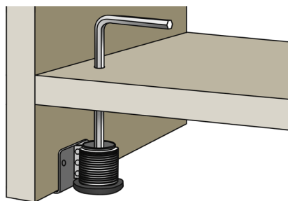
Скрытые регулируемые ножки
