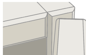
Обработка торцов кромкой 2 мм
